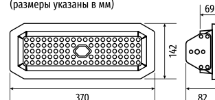
ДСП-112-00 75 Вт (размеры указаны в мм)
