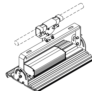
Тросовый подвес (до Ø20 мм)
