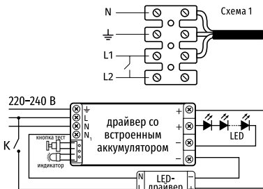
Схема подключения БАП в светильнике ДВО-19-А
