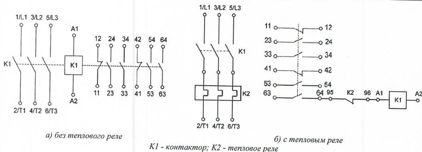
Рисунок 2. Принципиальная электрическая схема пускателя
