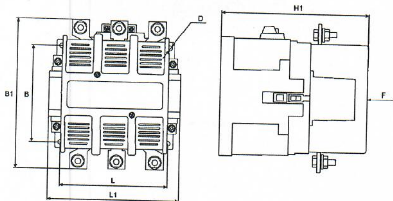
Рисунок 1. Пускатель неперевсивный ПМ12 315-1250А, IP00
