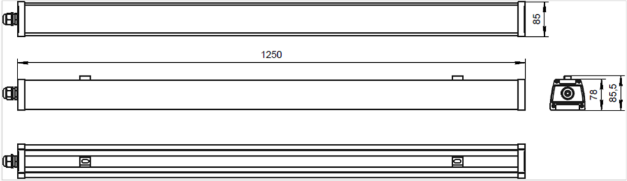
Рис. №5 Габаритный чертёж.
