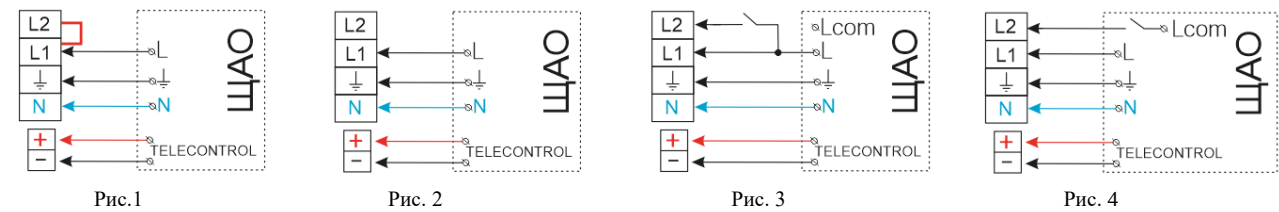
Рис. №1, 2, 3, 4 Схема подключения к групповой цепи питания и управления.
