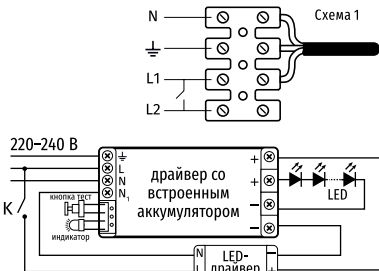
Схема подключения БАП в светильнике ДВО-16-А
