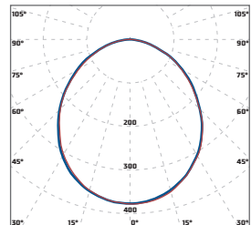
«Diora Office Glass opal » косинусная КСС 105°
