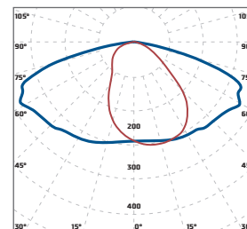
«Diora Unit PRO Ш4» широкая боковая КСС 150°x75°
