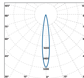
«Diora Unit К14» концентрированная КСС 14°
