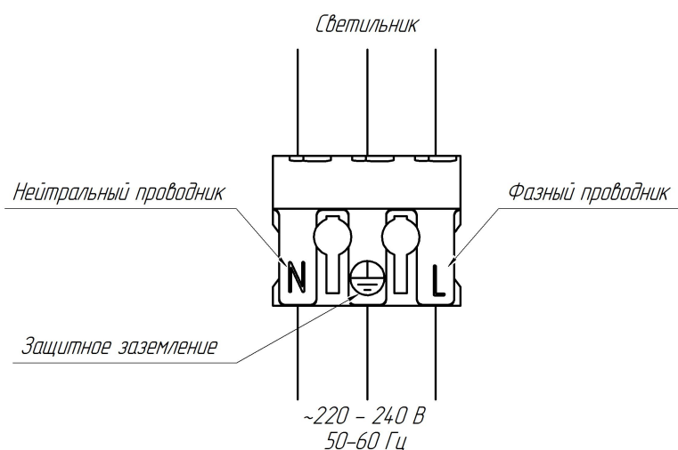
Рис. 2 Схема подключения.
