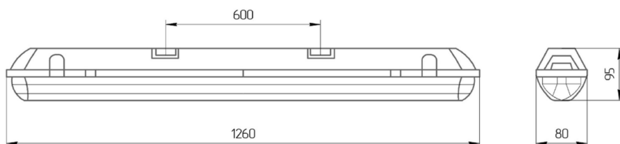
Рис. 1 Габаритный чертеж.
