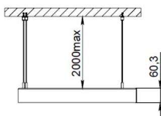
Рис.1 Габаритный чертеж.
