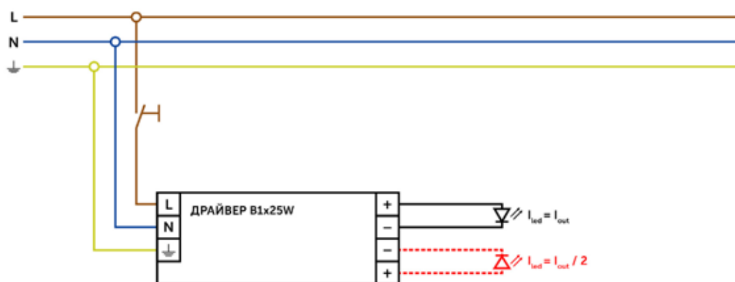
СХЕМА ПОДКЛЮЧЕНИЯ ДЛЯ ДРАЙВЕРА LT B1x25W
