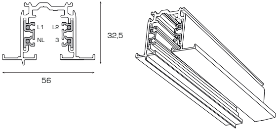
Встраиваемый трехфазный шинопровод
