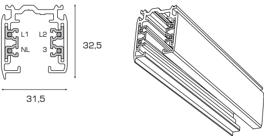
Подвесной/накладной трехфазный шинопровод
