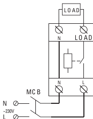
Рис. 8 - Условная схема подключения
