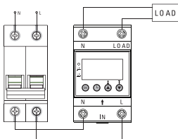
Рис. 9 - Схема подключения
