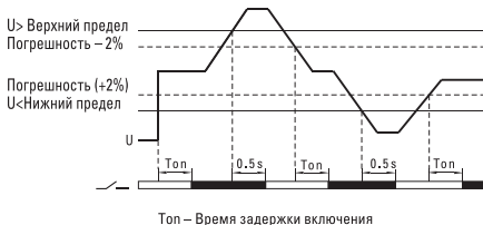
Рис. 1 - Диаграмма работы реле
