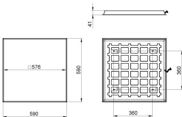
Рис.1 Габаритный чертеж.
