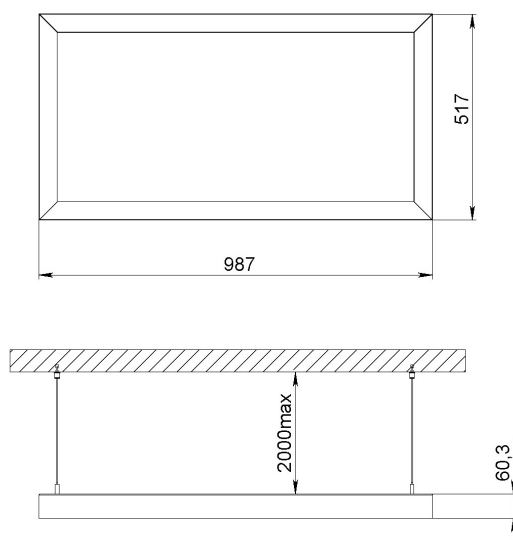
Рис.1 Габаритный чертеж.
