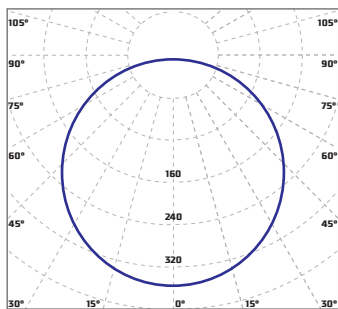
«Diora NPO [NPO Mini] IP65 opal» косинусная КСС 110°
