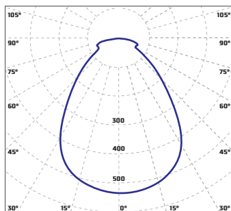
«Diora NPO [NPO Mini] IP65 microprism» косинусная КСС 80°
