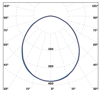
«Diora NPO [NPO Mini] Glass» косинусная КСС 100°
