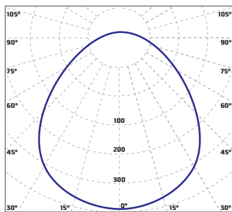
«Diora NPO [NPO Mini] IP65 prism» косинусная КСС 90°
